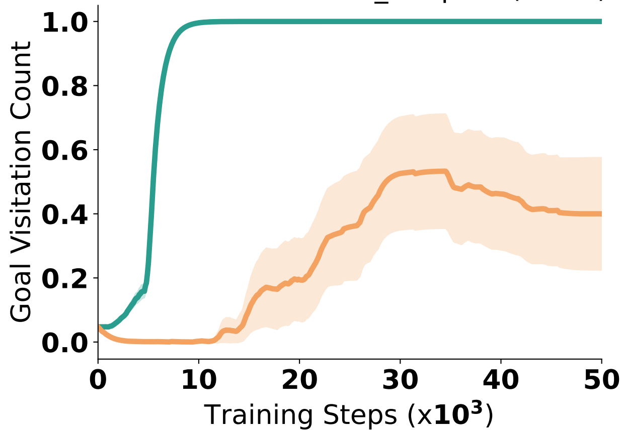
Gridworld-Bottleneck_NExperts(100%)
